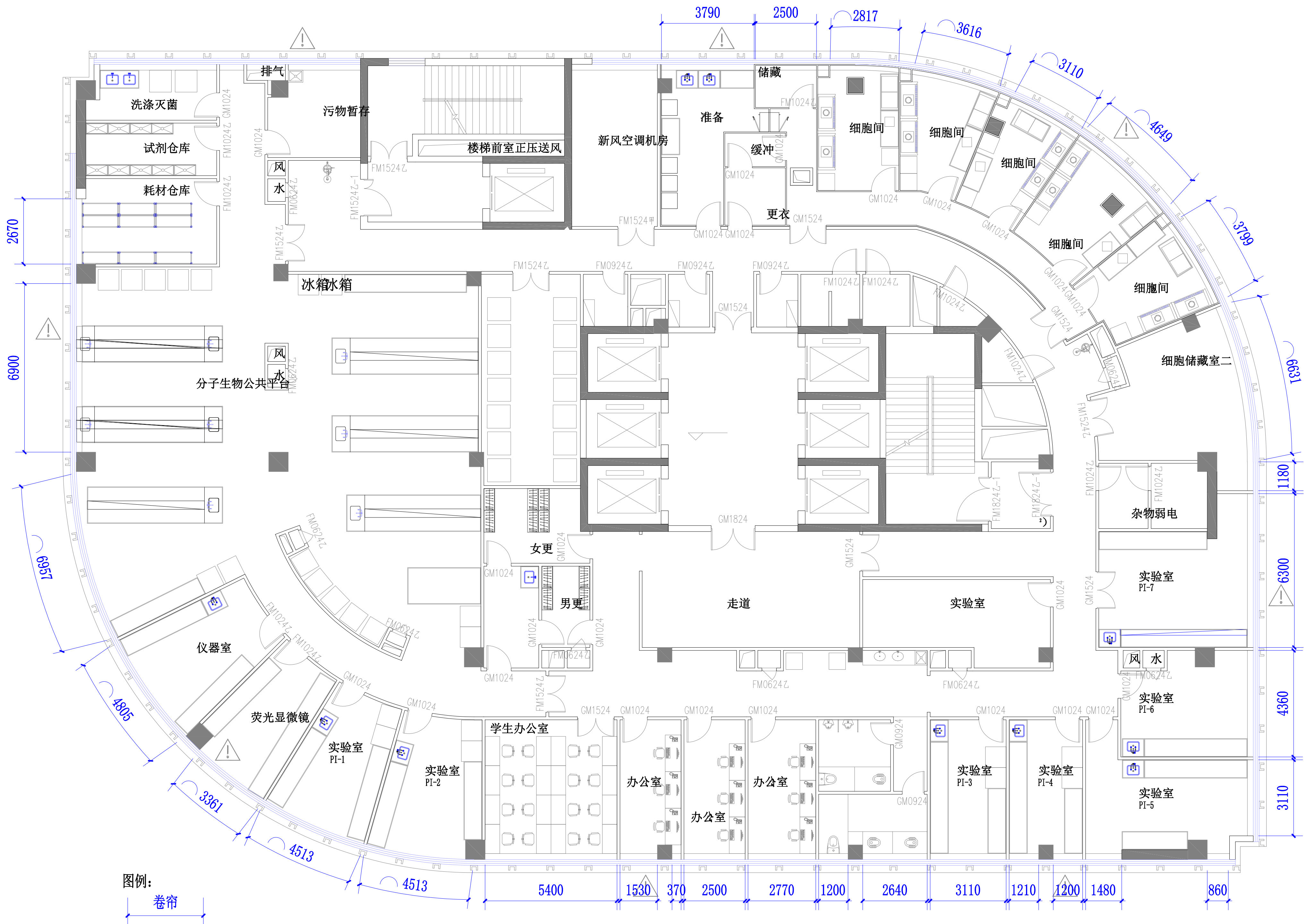
十二层平面布置图
