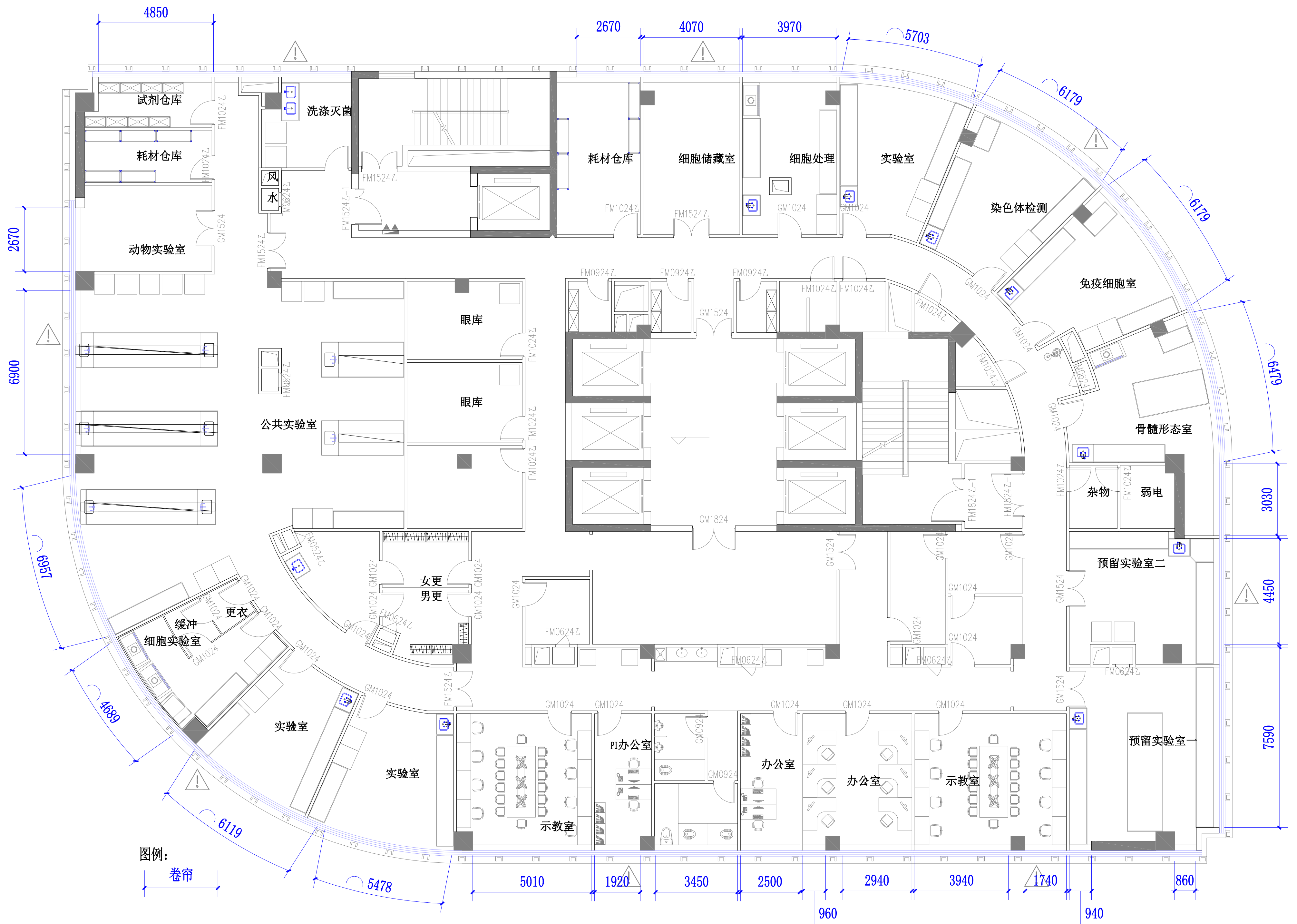
十一层平面布置图
